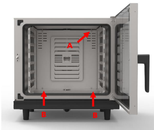
Figura 49. Tornillos de fijación de la chapa de aspiración para COOK PRO
