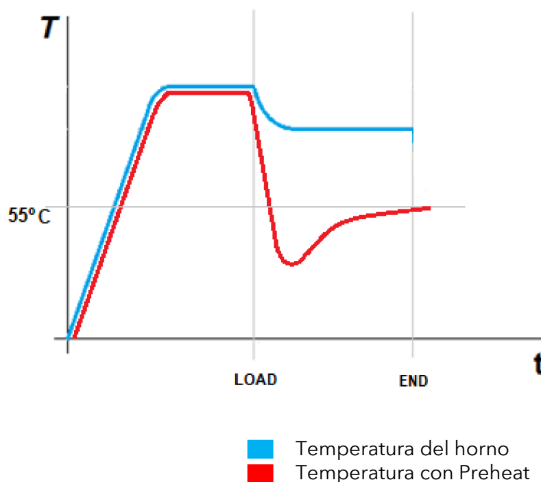
Figura 19. Evolución de temperatura con Preheat y sonda
